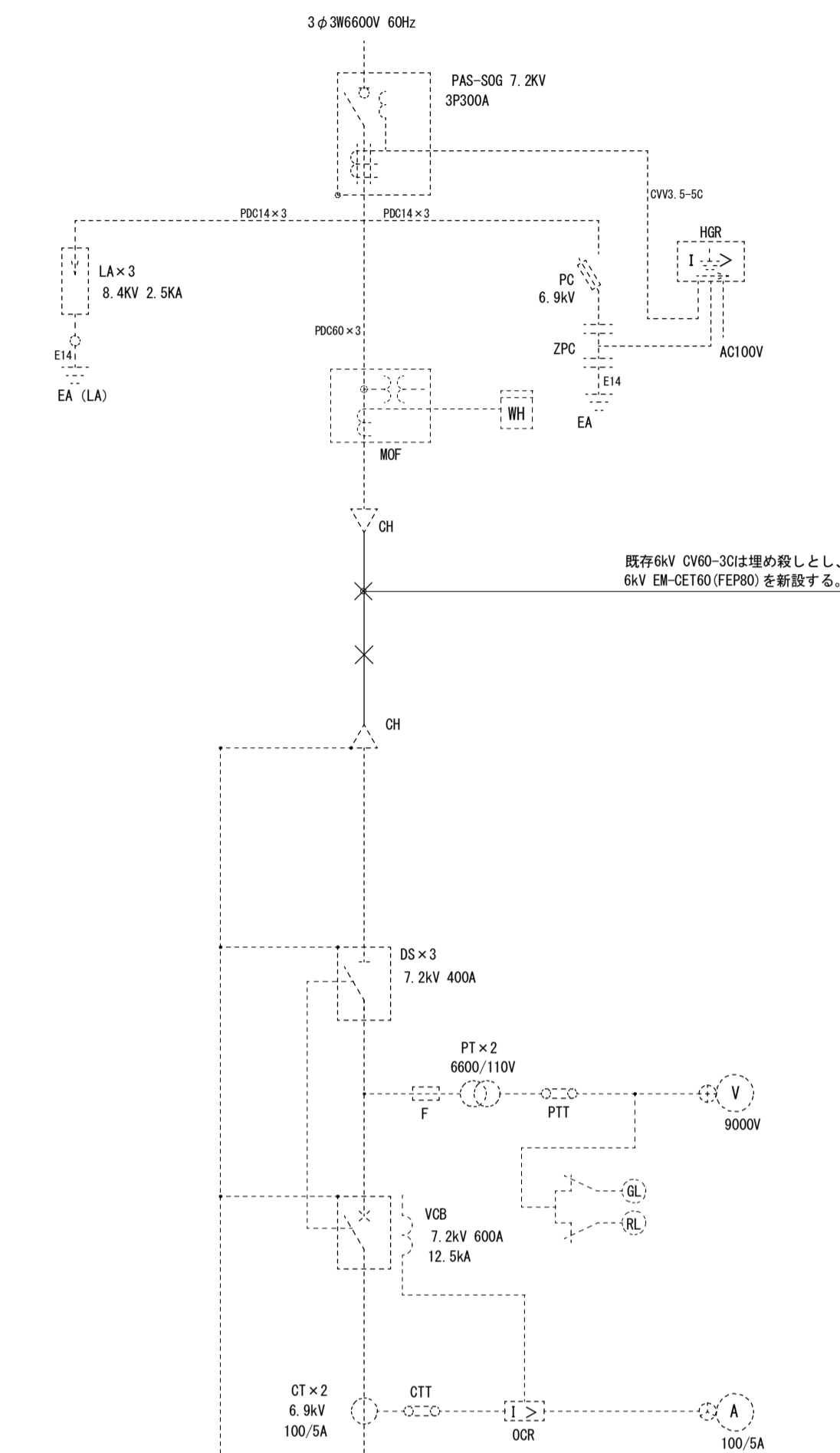
高圧受電設備単線結線図
