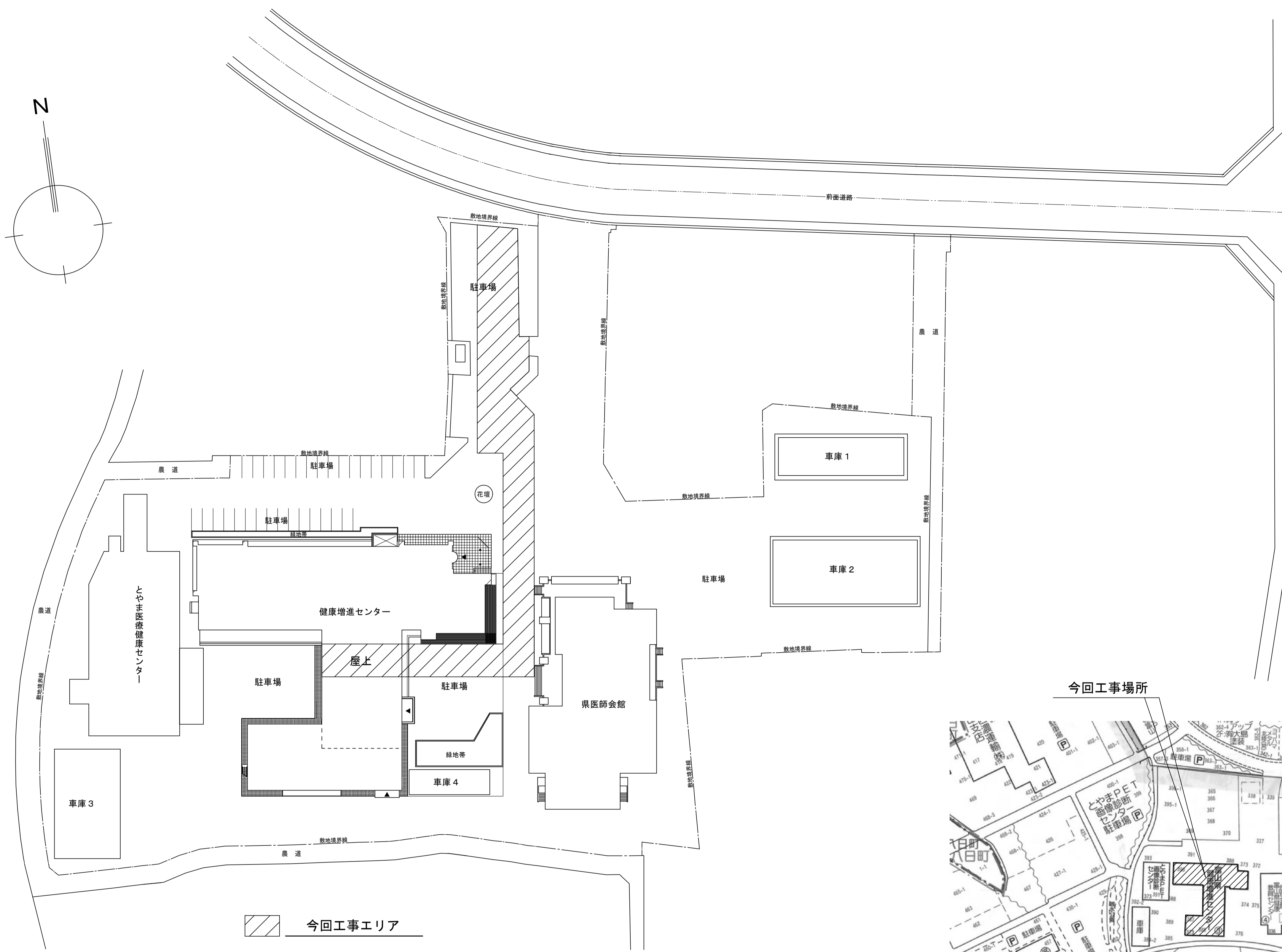
敷地配置図 1:500
